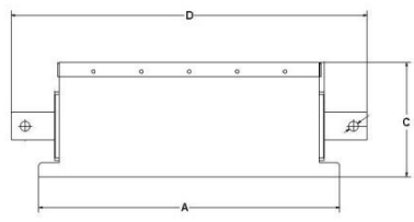
Fig 1 (Busbar type)
